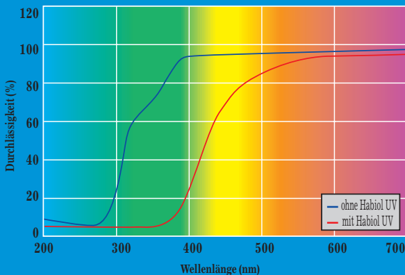
Lichtdurchlässigkeitskurven mit Habiol UV
